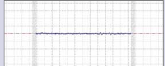
Nach Microfinish
